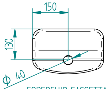
COPERCHIO CASSETTA
