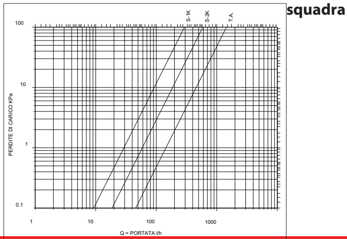
squadra 3/8" - 1/2" QmN 185
