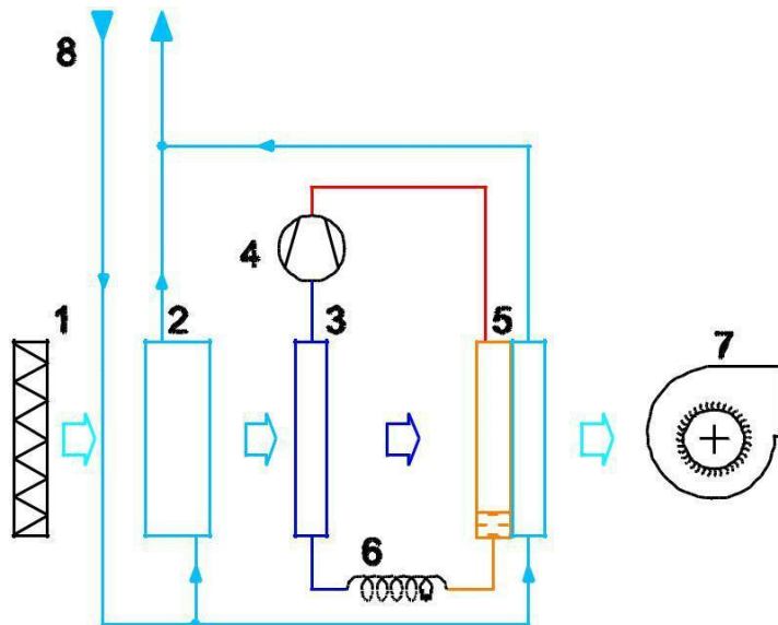
Fig. 1 Schema del deumidificatore ENERGY E24
