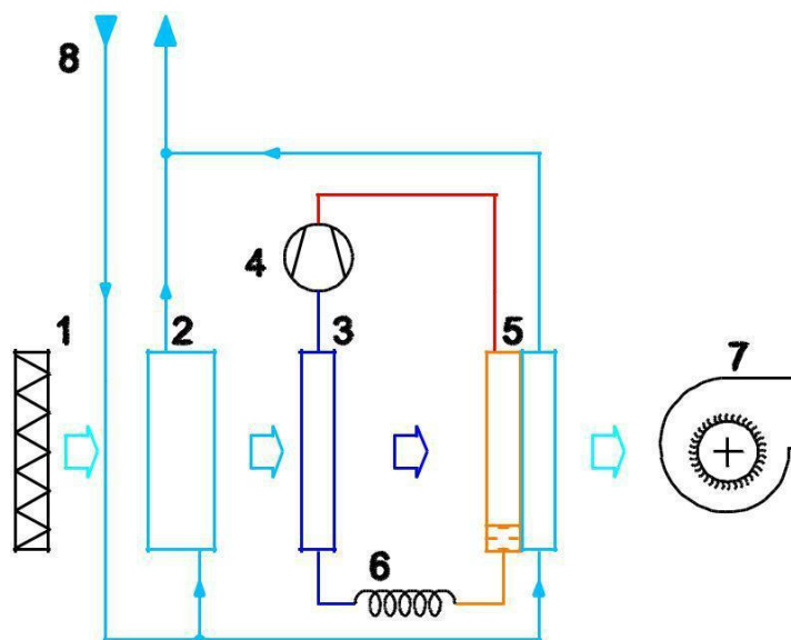
Fig. 1 Schema del deumidificatore ENERGY E26
